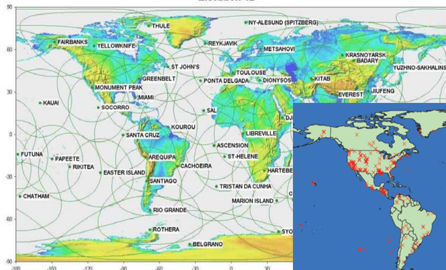
DORIS
