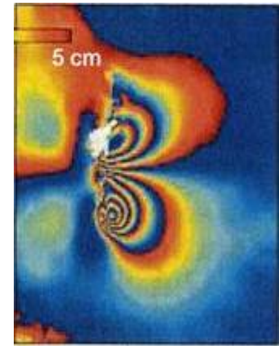
InSAR
